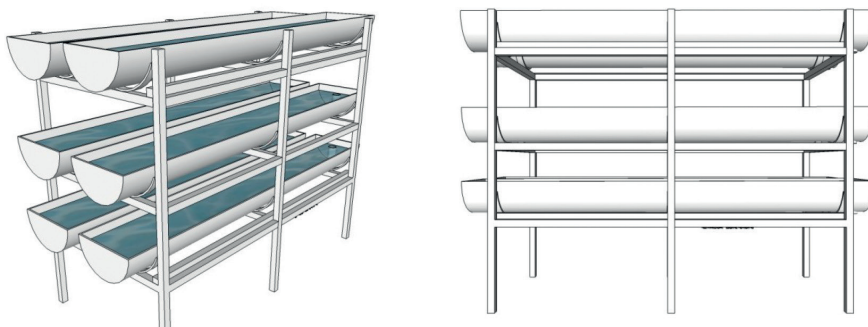
FIG. 24. Canaletas de plástico PVC para mantenimiento de larvas.
