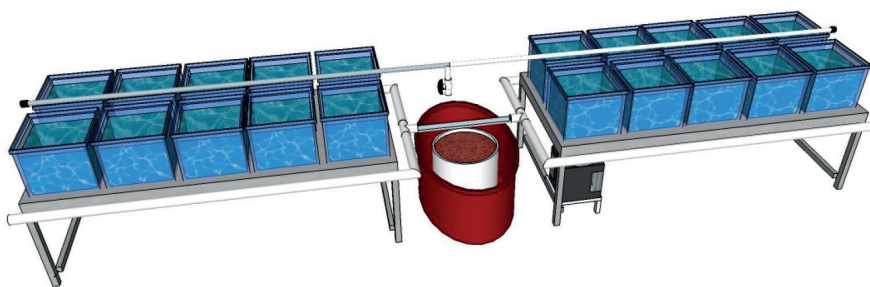
FIG. 23. Sistema de tinas en sistema para cultivo de larvas de pescado blanco.
