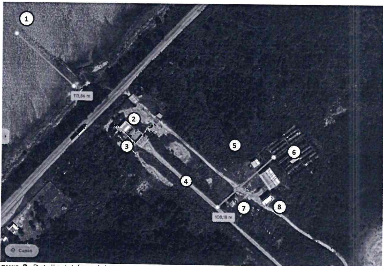
Figura 2. Detalle del área del proyecto: 1) Toma de agua de mar, 2) Área de bombeo, 3) Reservorio, 4) Canal de llamada, 5) Pozo, 6) Zona de raceways, 7) Laboratorio, y 8) bodega de alimento y dormitorios.
