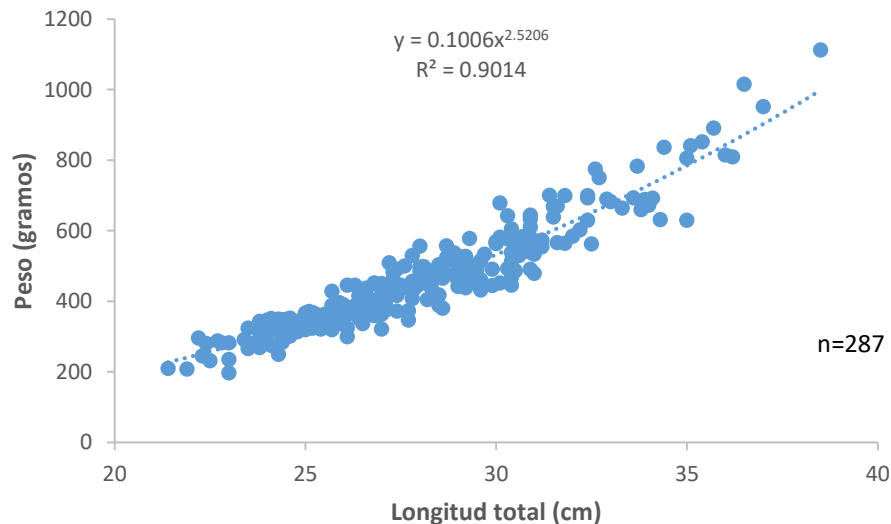
Figura 2.- Correlación longitud total-peso de Oreochromis spp .
