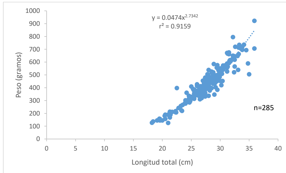
Figura 2.- Correlación longitud total-peso de Oreochromis sp.
