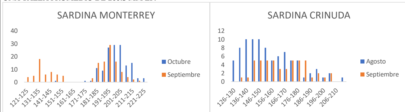
FIGURA 1: DISTRIBUCION DE FRECUENCIA DE TALLAS DE LA SARDINA MONTERREY Y SARDINA CRINUDA EN BAHÍA MAGDALENA DURANTE LOS MESES DE AGOSTO SEPTIEMBRE Y OCTUBRE DEL 2024.
