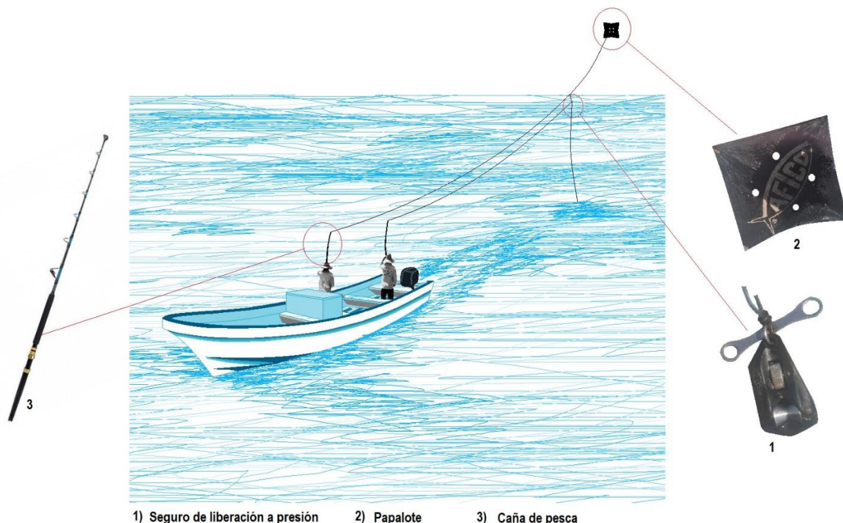
Figura 1. Forma de operación y partes principales que componen la pesca de atún con papalote
