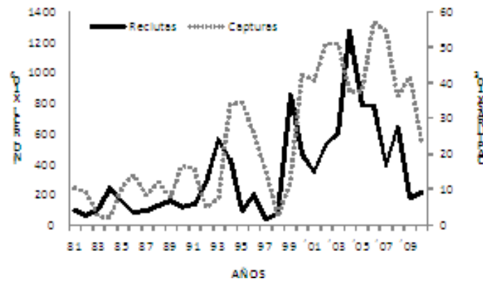
Figura 24.- Índice de abundancia de las clases anuales de sardina monterrey en Bahía Magdalena, B.C.S. (actualizado de Félix-Uraga et al., 2004).
