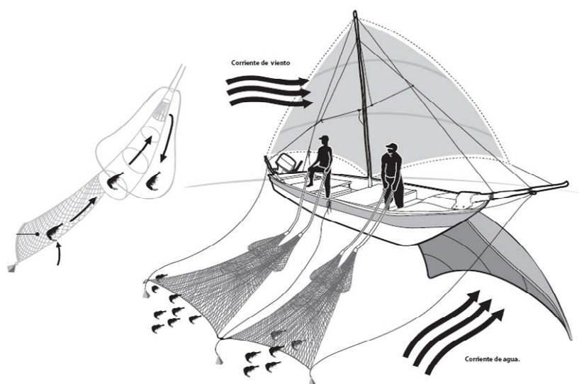
Esquema de las atarrayas “Suripera”, demostrando su principio operativo
