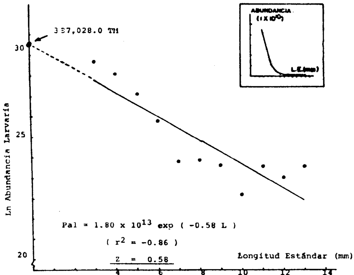
Figura 11. El Ajuste con la Función Exponencial provee una Estimación del Coeficiente Instantáneo de Mortalidad ( Z ), por mm de Longitud Estándar. En el recuadro se presenta la forma funcional de los valores de abundancia respecto a la talla.
